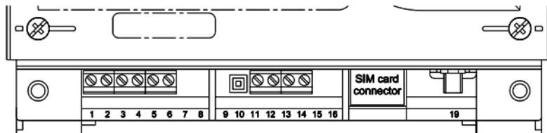
в) обозначение контактов счетчика СЕ303 S3x для исполнений со встроенным GSM-модулем
