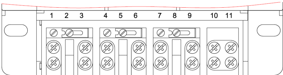
д) - обозначение контактов зажимов счетчика CE303 S31 74X
